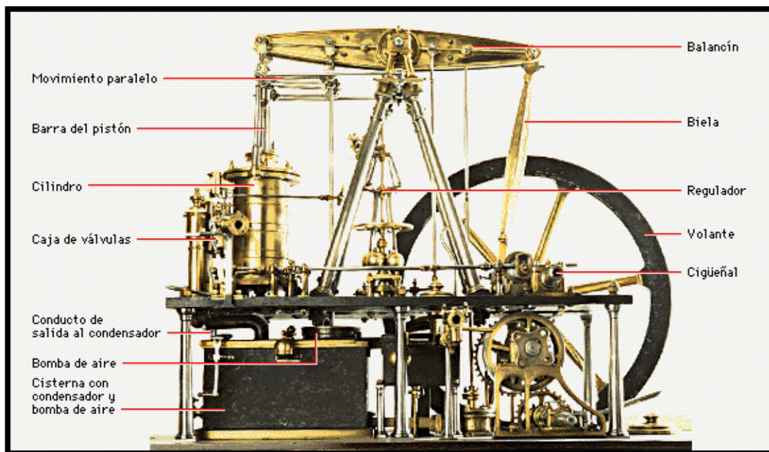
Máquina de vapor
