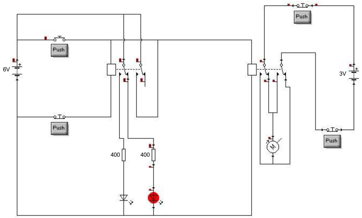
Ascensor.ckt
